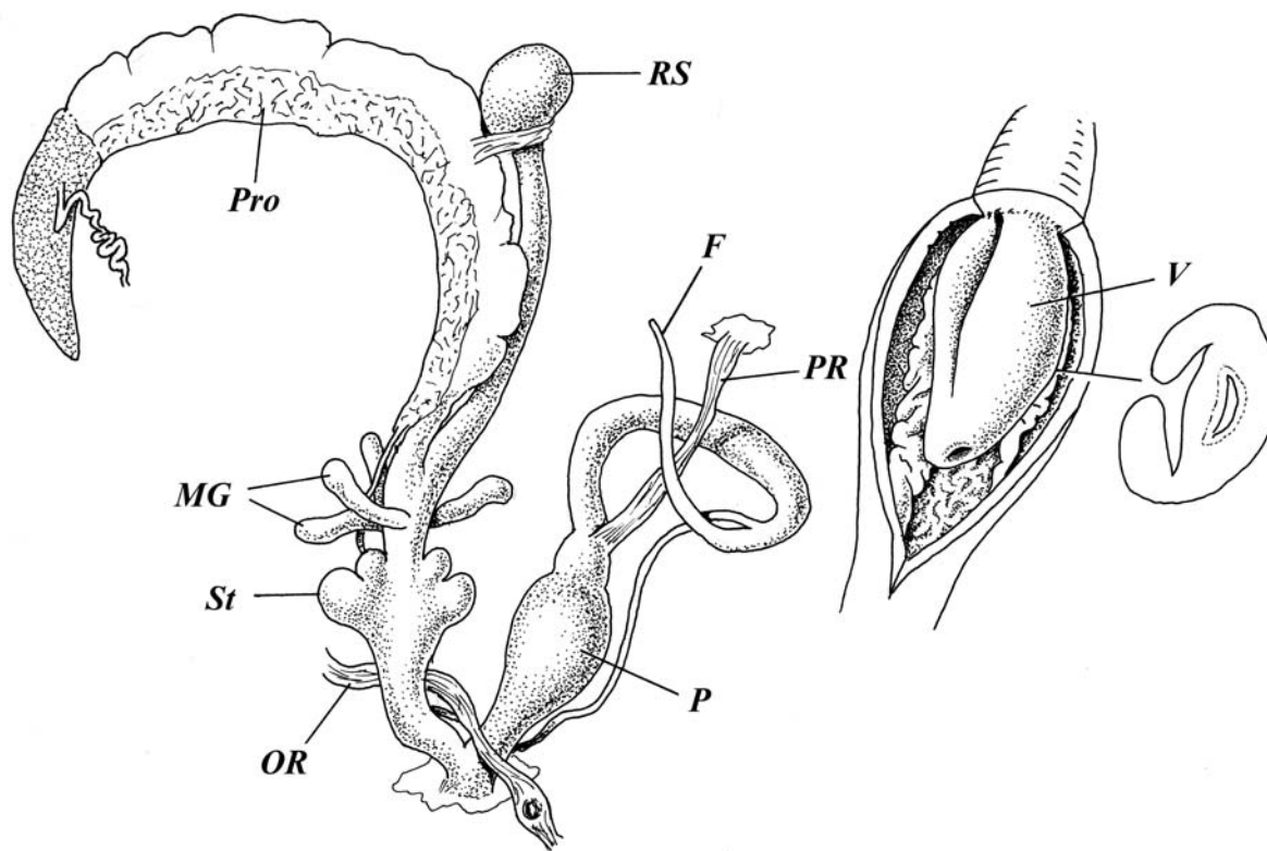
РИС. 3. Leucozonella corona sp. nov. Паратип. Репродуктивный тракт и внутреннее строение пениса. F — флагеллум, MG — слизистые железы, OR — ретрактор омматофора, P — пенис, PR — ретрактор пениса, Pro — простата, RS — резервуар семеприемника, St — стилофор, V — папилла пениса.
