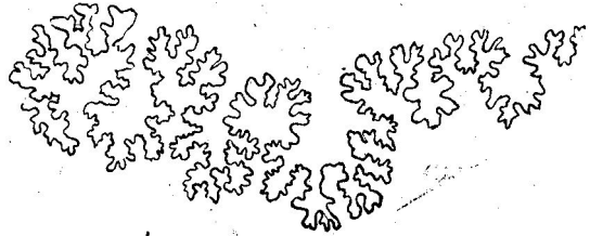
Рис. 14. Часть лопастной линіи Placenticeras kharesmense Lahusen. 1 / 1 . Видны полностью пять первыхъ сѣделъ и половина шестого.
