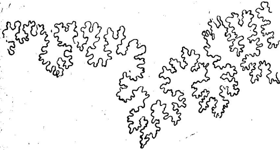
Рис. 13. Часть лопастной линіи Placenticeras kharesmense Lahusen. 1 / 1 . Отъ первого сѣдла видна лишь небольшая часть.
