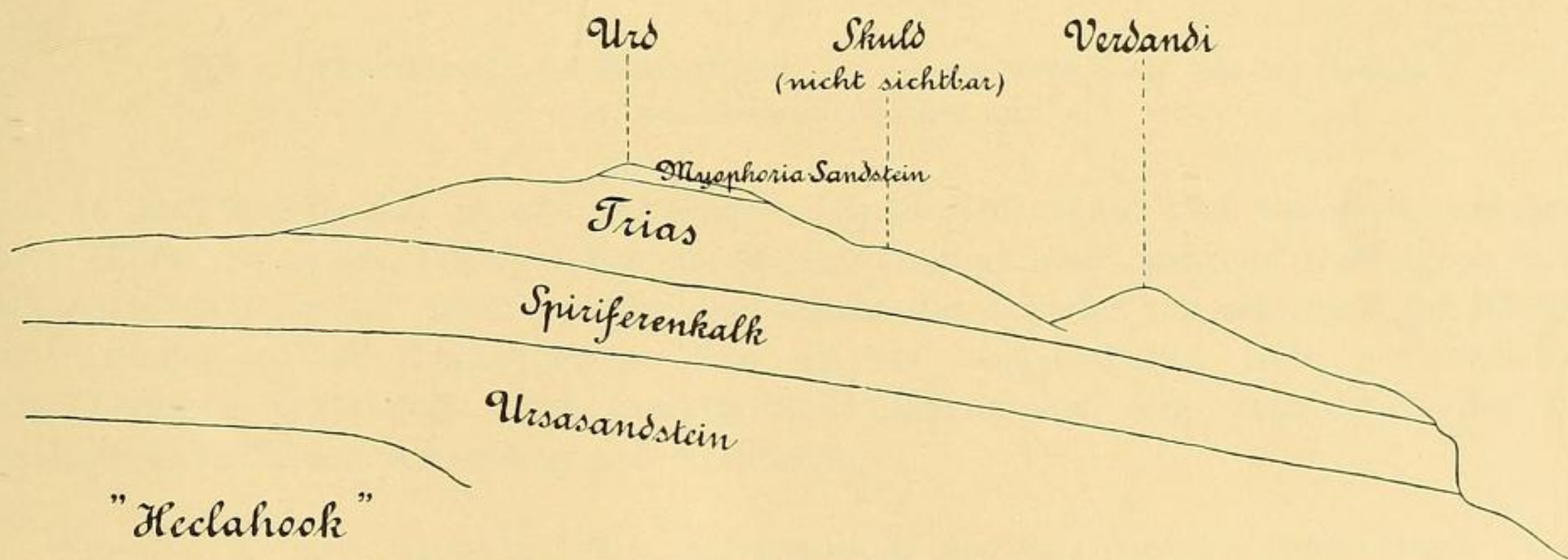
Fig. 2. Die geologische Reihenfolge des Mount Misery.
