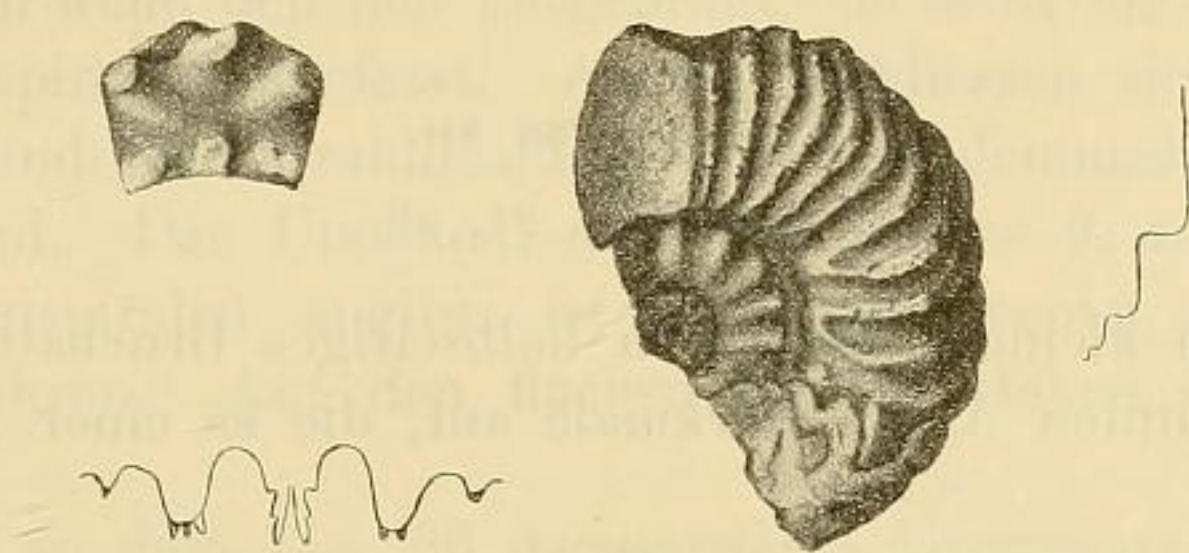
Fig. 9. Clionites Barentsi n. sp.
