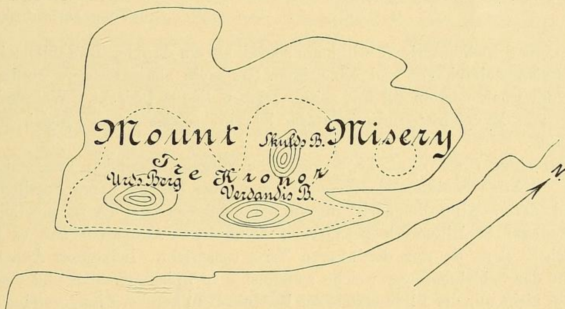
Fig. 3. Planzeichnung des Mount Misery. — Die punktierte Linie gibt die Gebiete der mesozoischen Schichten an.
