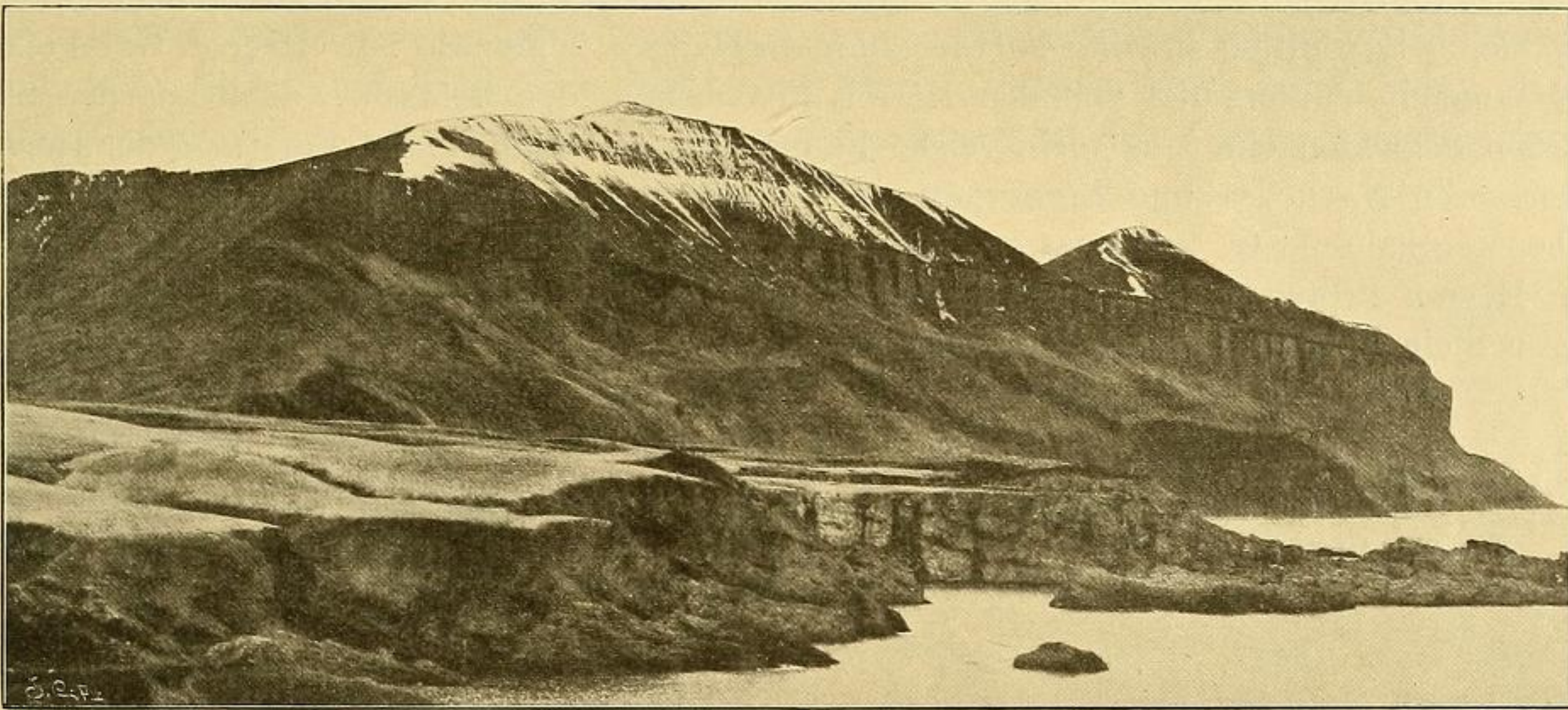
Fig. 1. Mount Misery, vom Russenhafen gesehen. (Phot. von J. G. ANDERSSON.)
