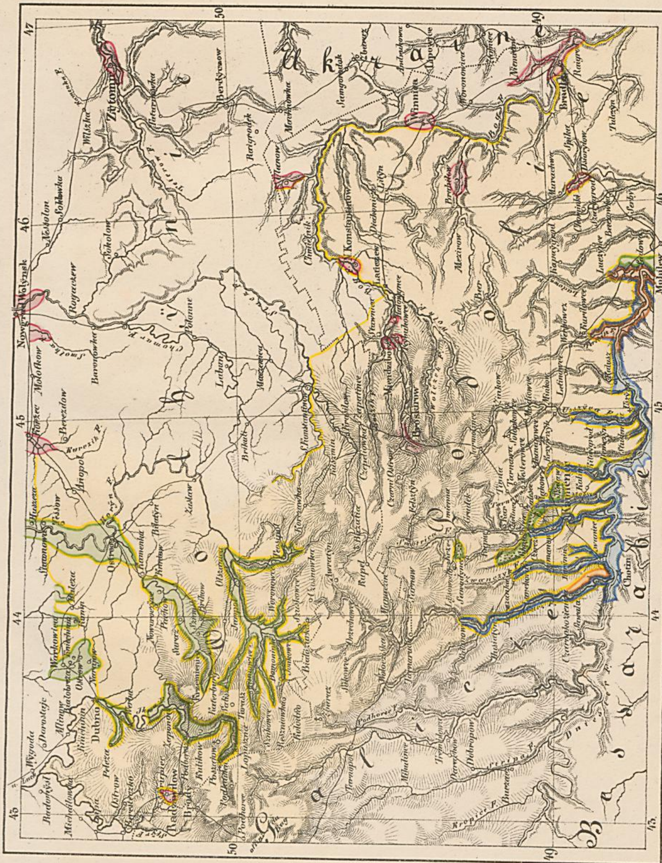
Plateau Wollyni - Podolien. granit. Massifs. Calcaires. Gyps. Strat. quatern.
